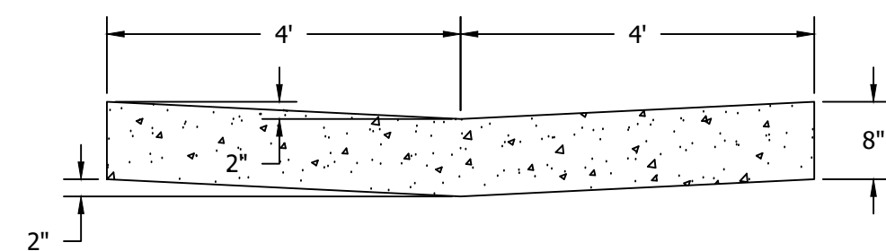
SECTION A-A
