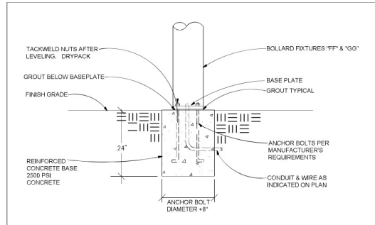
2 TYPES "FF" & "GG" POLE BASE DETAIL SCALE: N.T.S.
